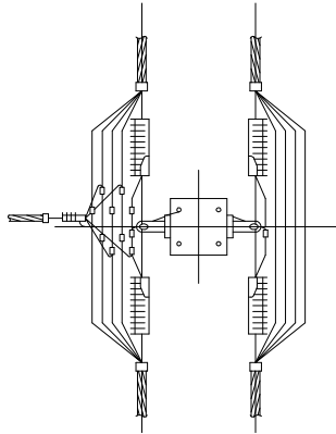
Схема ответвления к входу в здания в одну сторону 4х жил СИП
