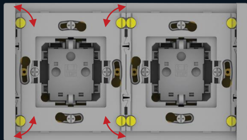
Эксцентрики для регулировки зазоров между механизмами
