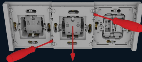
Пазы под отвёртку для извлечения суппорта из ряда
