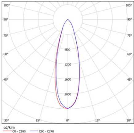
Исполнение «К15»
