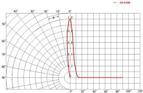
Исполнение «К15»
