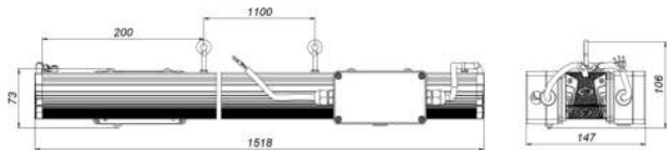
Рисунок 2 Светильник «L-fusion Office/Em» 1,5 м
