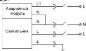
Рисунок 3 Схема подключения светильника
