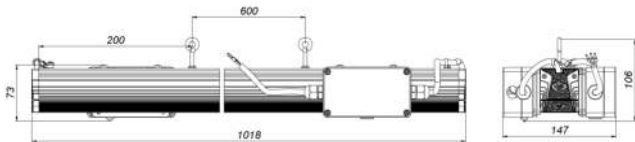
Рисунок 1 Светильник «L-fusion Office/Em» 1,0 м
