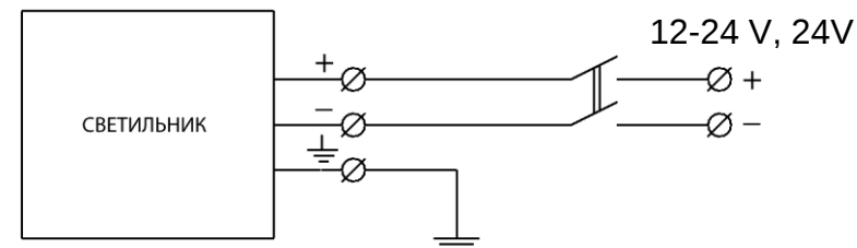
Рисунок 2 Схема подключения светильника
