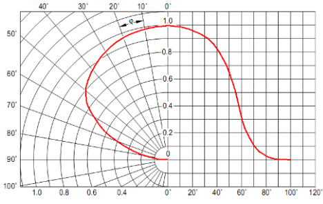
Рисунок 3 Тип КСС
