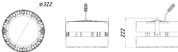
Рисунок 1 Общий вид светильника L-industry II Pro.
