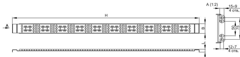
Рисунок / Figure 3 – Внешний вид органайзера кабельного вертикального / Appearance of the vertical cable organizer
