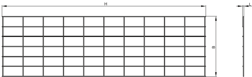
Рисунок / Figure 6 – Внешний вид органайзера кабельного горизонтального проволочного 300 / Appearance of the 300 horizontal wire-mesh cable organizer
