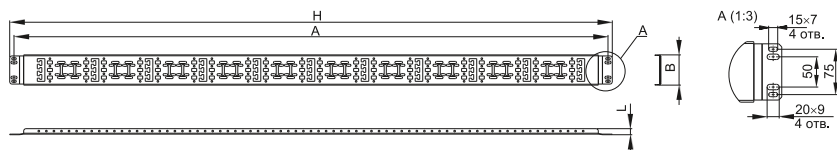
Рисунок / Figure 1 – Внешний вид органайзера кабельного вертикального 800 / Appearance of the 800 vertical cable organizer
