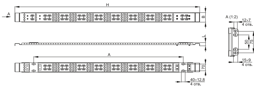
Рисунок / Figure 7 – Внешний вид органайзера кабельного вертикального для блока розеток / Appearance of vertical cable organizer for PDU
