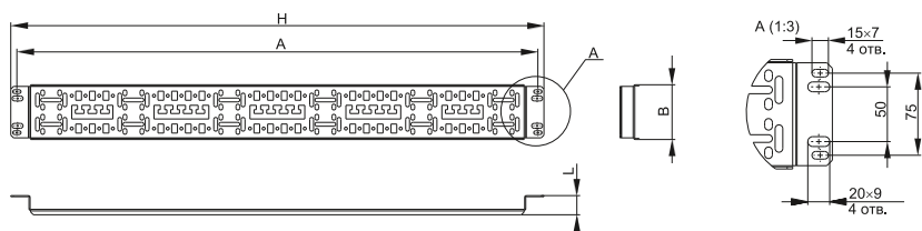
Рисунок / Figure 4 – Внешний вид органайзера кабельного горизонтального / Appearance of the horizontal cable organizer
