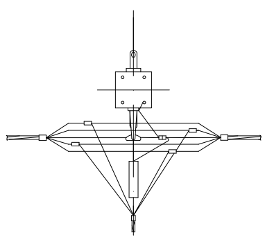
Схема ответвления к вводу в здания
