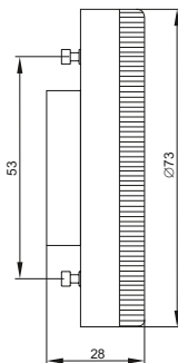
Рисунок 18 – Лампа LED T75, 12 Вт, 15 Вт, цоколь GX53
