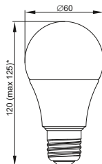
* Изготавливается в двух исполнениях по габаритным размерам Рисунок 4 – Лампа LED A60, 20 Вт цоколь E27
