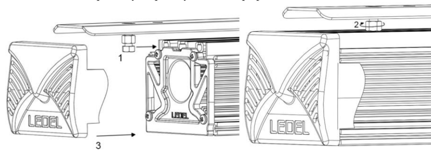
Рисунок 6 Схема монтажа подвешного крепления светильника
