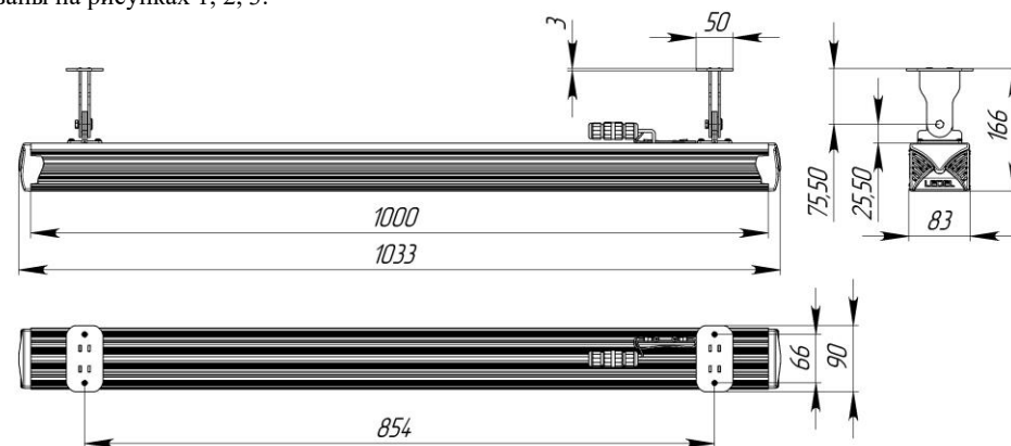
Рисунок 1 Светильник «L-industry NEW 48». Поворотный вариант
