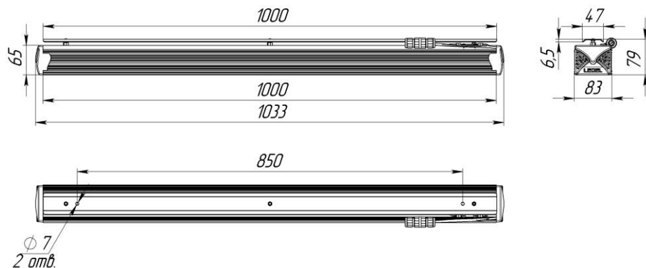
Рисунок 3 Светильник «L-industry NEW 48». Задвижной вариант
