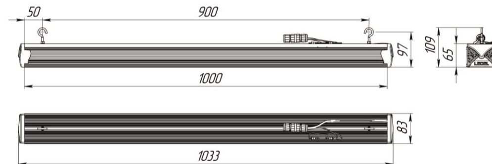
Рисунок 2 Светильник «L-industry NEW 48». Подвесной вариант
