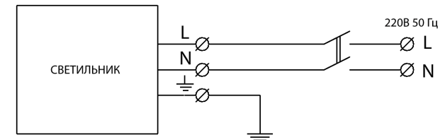
Рисунок 4 Схема подключения светильника
