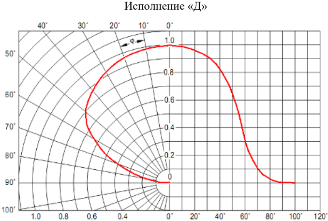
Рисунок 13 Тип КСС
