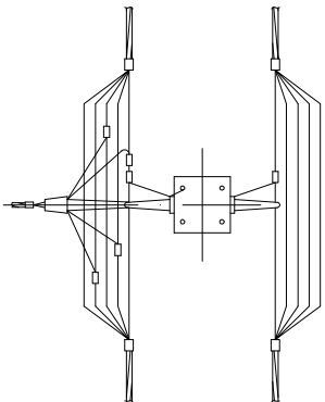
Схемы отметвления к входу в здания в одну сторону 4* жил СИП
