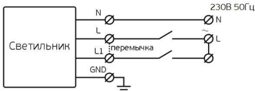
Рисунок 2 Схема подключения светильника
