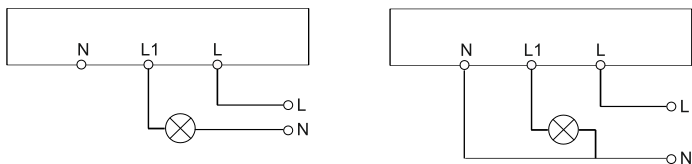
Рисунок 2 – Электрические схемы подключения датчика движения
