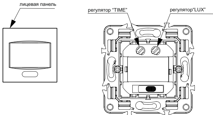
Рисунок 1 – Конструкция датчика движения
