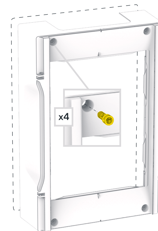
1.7 Крепление крышки к основанию Mount of the cover to the base
