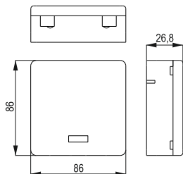
Рисунок 1 – Розетка оптическая настенная 2 порта SC/LC
