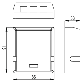
Рисунок 3 – Розетка мультимедиа настенная 3 порта SC/LC KJ
