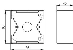
Рисунок 4 – монтажная коробка для розеток
