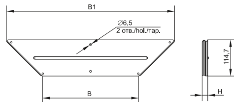
Рисунок / Figure / Сурет 3 – Крышка отвода Т-образного 1,2; 1,5 мм / Cover of T-branch 1,2; 1,5 mm / Т-тәрізді бұру қақпағы 1,2; 1,5 мм
