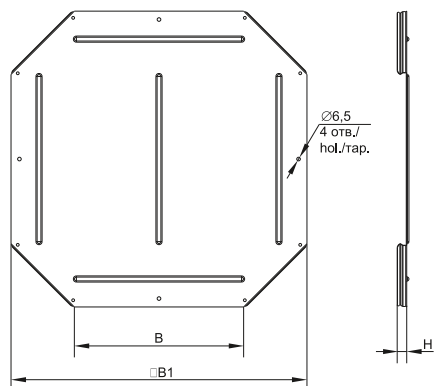
Рисунок / Figure / Сурет 7 – Крышка на крестовину 1,2; 1,5 мм / Cover of T-branch 1,2; 1,5 мм / Айқастырма қақпағы crossover 1,2; 1,5 мм
