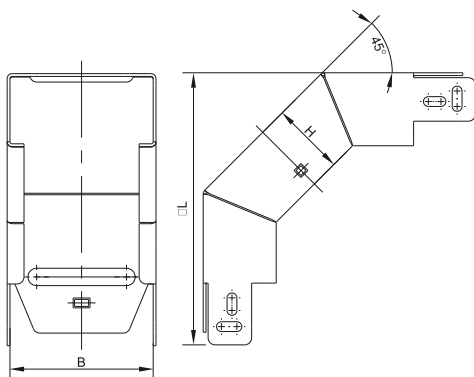
Рисунок / Figure / Сурет 26 – Поворот вертикальный внутренний 90 град. 2,0 мм / 90° vertical internal bend 2,0 mm / Ішкі тік бұрылыс 90 градус 2,0 мм
