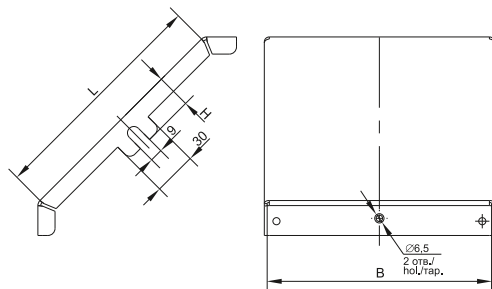
Рисунок / Figure / Сурет 24 – Крышка поворота вертикального внешнего 90 град, 2,0 мм / Cover of 90° vertical external bend 2,0 mm / Қақпақтың сыртқы тік бұрылысы 90 градус 2,0 мм
