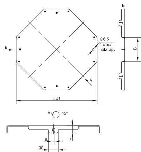
Рисунок / Figure / Сурет 7 – Крышка на крестовину 1,2; 1,5 мм / Cover of T-branch 1,2; 1,5 мм / Айқастырма қақпағы crossover 1,2; 1,5 мм
