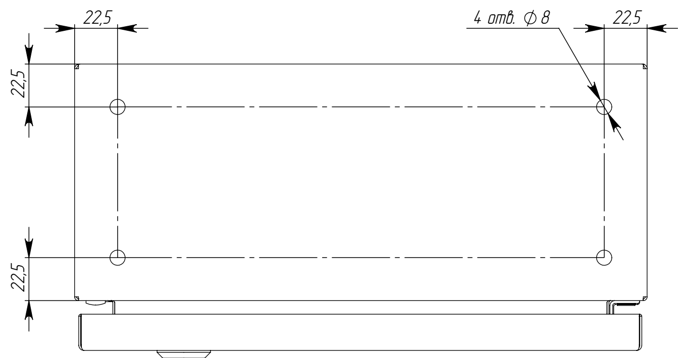
Разметка отверстий для установки козырька
