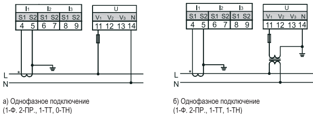
Рисунок 2 — Схема подключения анализатора качества электроэнергии PQ720, PQ720C серии ARMAT (лист 1 из 3)
