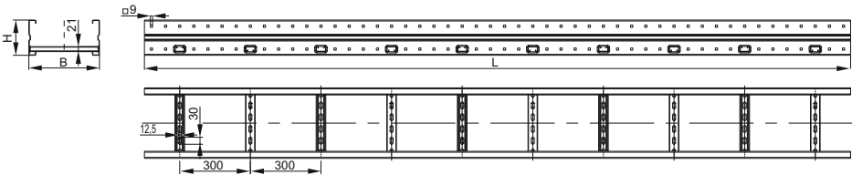
Рисунок 1 – Лоток лестничный LESTA 5H / Figure 1 – Ladder tray LESTA 5H / 1-сұрет – LESTA 5H сатылы науасы
