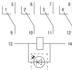
Блок светодиодной индикации / LED indication unit / Жарық диодты индикациялау блогы
