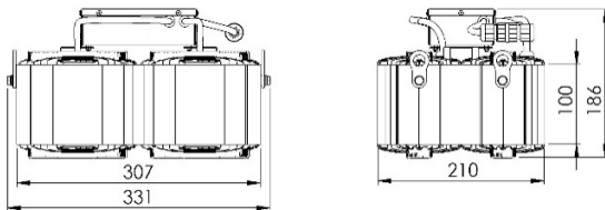
Рисунок 1 Общий вид светильника «L-lego II 220» Подвесное крепление
