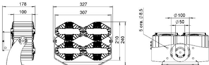
Рисунок 2 Общий вид светильника «L-lego II 220 banner» Поворотное крепление
