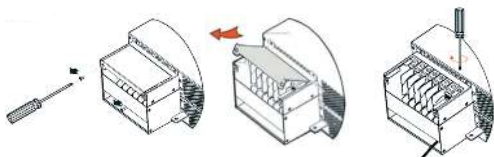
Рисунок 71 – Демонтаж защитной крышки контактов ИБП типа MPOR120
