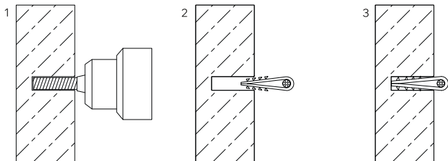
Рисунок 3 – Порядок монтажа хомута
