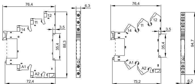
а) IMR-470-UT-1-SOC-U024-0LV; IMR-470-UT-1-SOC-U220-0LV
