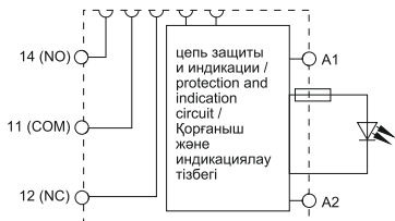
Рисунок 2 – Схема электрическая розетки / Figure 2 – Electrical diagram of the socket / 2 сурет – Розетканың электрлі схемасы
