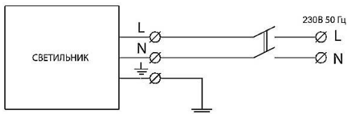
Рисунок 6 Схема подключения светильника
