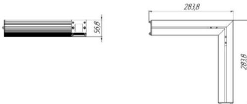
Рисунок 3 Светильник «L-fusion Office MG L
