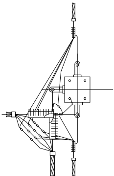
Схема отведений к вводу в здания в две стороны 4х жил СИП
