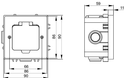
Рисунок 1 – Лючок в бетонный пол / Figure 1 – Box into concrete floor / 1 сурет – Бетон еденнің ойымшасы (PM-LN43-02-O-44-KXX)
