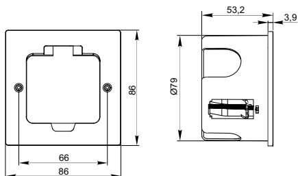
Рисунок 2 – Лючок в фальшпол / Figure 2 – Box into raised floor / 2 сурет – Жалған еденнің ойымшасы (PM-LN33-02-O-44-KXX)
