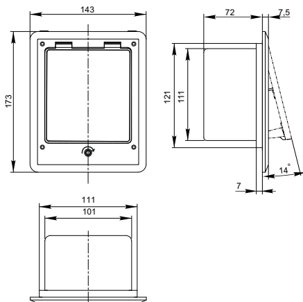
Рисунок 5 – Лючок напольный с ключом на 3 или 6 модулей / Figure 5 – Floor box with key lock for 3 or 6 modules / 5 сурет – 3 не 6 модульдік кілтті еден ойымшасы (PM-LN12-03-K-66-KXX, PM-LN12-06-K-66-KXX)
