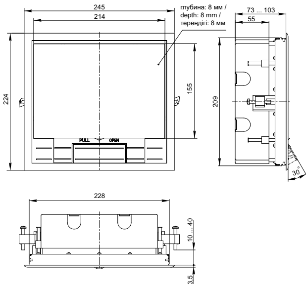
Рисунок 8 – Лючок напольный 12 модулей / Figure 8 – Floor box 12 modules / 8 сурет – 12 модульдік еден ойымшасы (PM-LN12-12-O-20-KXX, PM-LN14-12-O-20-KXX)
