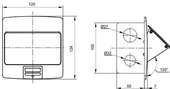
Рисунок 6 – Лючок с откидной крышкой на 3 модуля / Figure 6 – Hinged cover box for 3 modules / 6 сурет – 3 модульдік қайырмалы қақпағы бар ойымша (PM-LN21-03-O-42-KXX)
