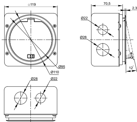
Рисунок 3 – Лючок круглый на 3 модуля / Figure 3 – Round box for 3 modules / 3 сурет – 3 модульдік дөңгелек ойымша (PM-LN12-03-O-65-KXX)
