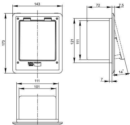
Рисунок 4 – Лючок напольный с кнопкой на 3 или 6 модулей / Figure 4 – Floor box with push button for 3 or 6 modules / 4 сурет – 3 не 6 модульдік түймешікті еден ойымшасы (PM-LN12-03-B-66-XX, PM-LN12-03-B-66-KXX)
