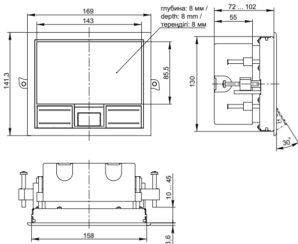
Рисунок 7 – Лючок напольный 8 модулей / Figure 7 – Floor box 8 modules / 7 сурет – 8 модульдік еден ойымшасы (PM-LN12-08-O-20-KXX)
