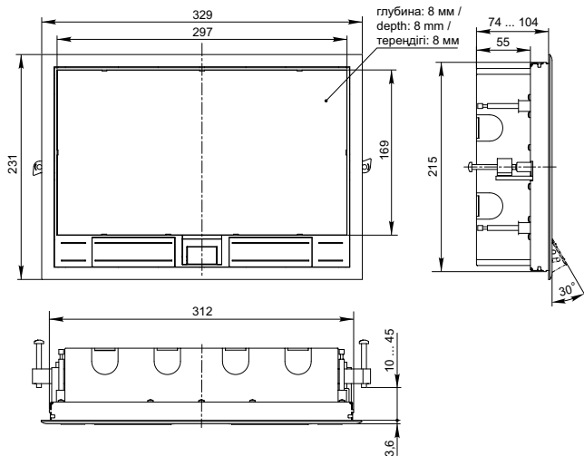
Рисунок 9 – Лючок напольный 16 или 24 модуля / Figure 9 – Floor box 16 or 24 modules / 9 сурет – 16 не 24 модульдік еден ойымшасы (PM-LN12-16-O-20-KXX, PM-LN12-24-O-20-KXX)
