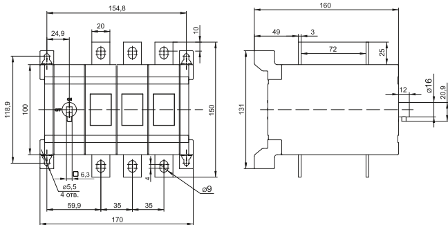
д) / i) БПК / VRK 160A-250A (реверсивный / reversible)
