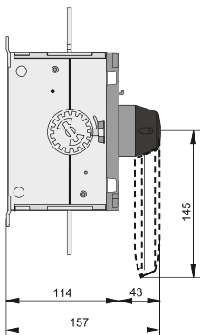
в) / c) BPK / VRK 630A – 800A
