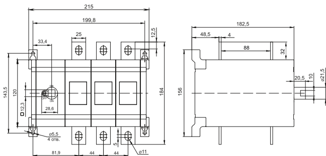
е) / f) БПК / VRK 315A-400A (реверсивный/ reversible)
