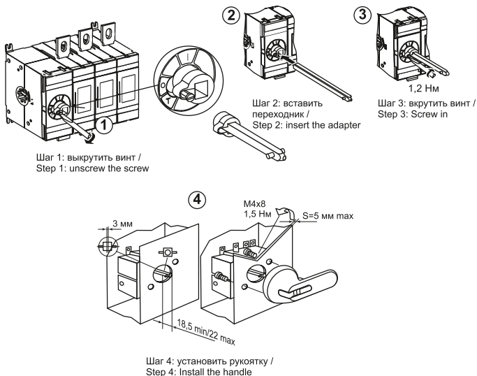
Рисунок / Figure 7 – Процедура монтажа ручки дистанционного управления / Installation procedure of the remote control handle
