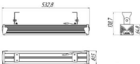
Рисунок 1 Светильник «L-industry NEW 24 L Em». Поворотный вариант
