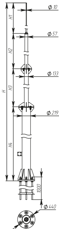
Рисунок / Figure / Сурет 8 – Мачта высотой 18000 мм / Air-termination mast 18000 mm high / Биіктігі 18000 мм діңгек
