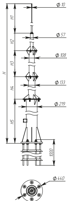
Рисунок / Figure / Сурет 9 – Мачта высотой 19500 мм / Air-termination mast 19500 mm high / Биіктігі 19500 мм діңгек
