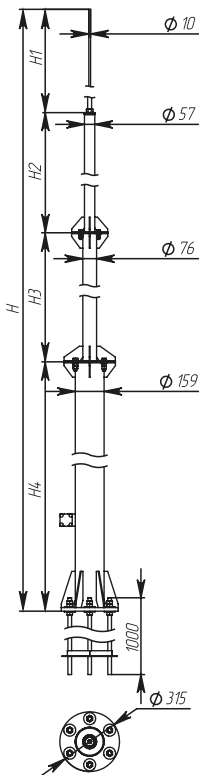
Рисунок / Figure / Сурет 5 – Мачта высотой 13500 мм / Air-termination mast 13500 mm high / Биіктігі 13500 мм діңгек
