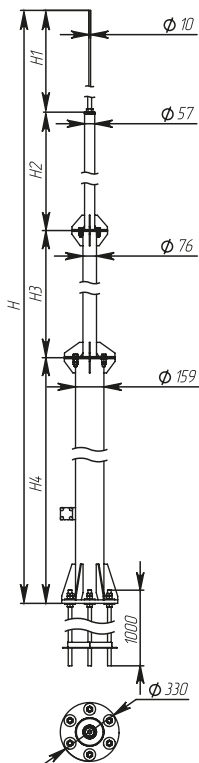
Рисунок / Figure / Сурет 6 – Мачта высотой 15000 мм / Air-termination mast 15000 mm high / Биіктігі 15000 мм діңгек
