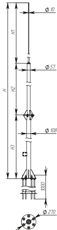
Рисунок / Figure / Сурет 4 – Мачта высотой 12000 мм / Air-termination mast 12000 mm high / Биіктігі 12000 мм діңгек
