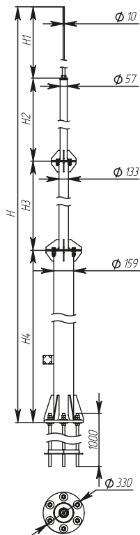
Рисунок / Figure / Сурет 7 – Мачта высотой 16500 мм / Air-termination mast 16500 mm high / Биіктігі 16500 мм діңгек
