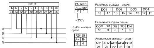
а) схема подключения мультиметра LED к четырехпроводной сети при I \leq 5 A, U \leq 600 В
