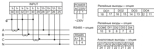
в) схема подключения мультиметра LED к четырехпроводной сети при I > 5 A, U \leq 600 В
