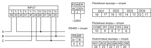
б) схема подключения мультиметра LED к трехпроводной сети при I \leq 5 A, U \leq 600 В
