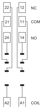
б) / b) IMR-470-ML-2-SOC-0000-0LV
