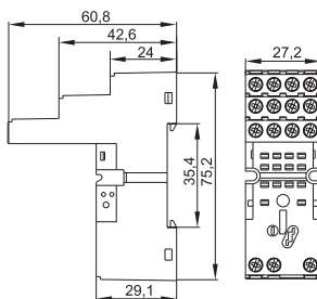
б) / b) IMR-470-ML-2-SOC-0000-0LV
