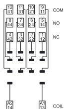
Рисунок 2 – Схемы электрические розетки / Figure 2 – Electrical diagrams of the socket / 2 сурет – Розетканың электрлі схемасы
