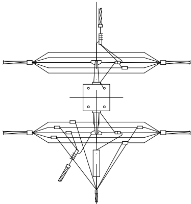
Схема отведений к вводу в здание в две стороны 2х жил СИП
