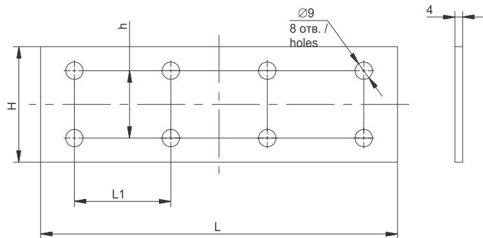
Рисунок / Figure 2 – Пластина соединительная / Joining plate
