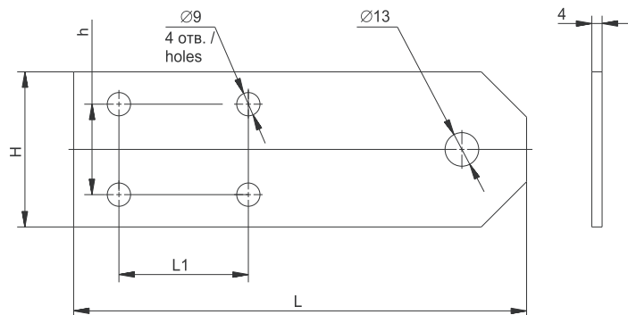
Рисунок / Figure 1 – Пластина шарнирного соединения / Hinge joint plate
