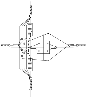
Схема ответвления к вводу в здания в две стороны 2х жил СИП
