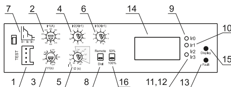
b) Типоразмер G, H, I / G, H, I frame sizes
