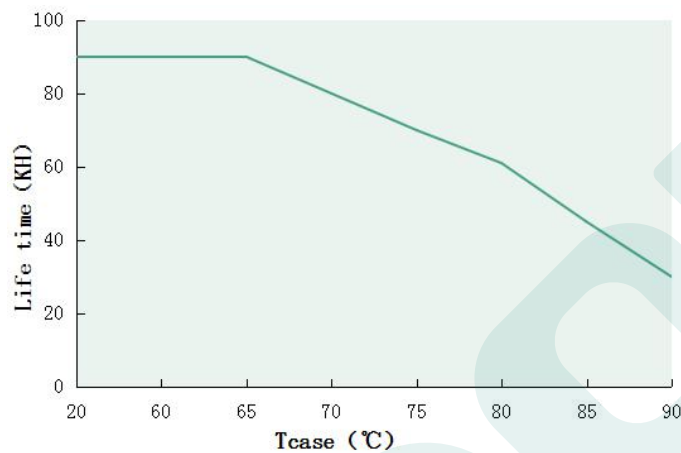
Tcase VS Lifetime(DL-75W-A/P/X-MXG)
