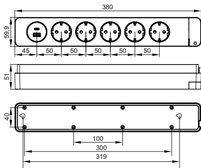
Удлинитель У05К / Cord extension set U05K / Ұзартқышы У05К
