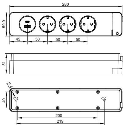
Рисунок 1 – Габаритные размеры удлинителей / Figure 1 – Overall dimensions of the extension sets / Сурет 1 – Ұзартқыштардың габариттік өлшемдері
