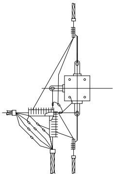
Схема ответвлений к вводу в здания в две стороны 2х жил СИП
