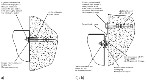
Рисунок / Figure / Сурет 2 – Крепление корпуса к стене / Mounting the enclosure to the wall / Корпусы қабырғаға бекіту
