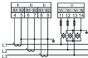
г) Трехфазное, трехпроводное подключение / Three-phase, three-wire connection / Yш фазалык, үш сымды жалғау (3P3W, 3-TT, 3-TN)
