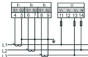
д) Трёхфазное, трёхпроводное подключение / Three-phase, three-wire connection / Үш фазалық, үш сымды жалғау (3P3W, 3-TT, 0-TH)
