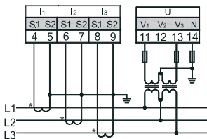
ф) Трёхфазное, трёхпроводное подключение / Three-phase, three-wire connection / Үш фазалық, үш сымды жалғау (3P3W, 3-TT, 2-TH)
