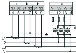
и) Трехфазное, четырехпроводное подключение / Three-phase, four-wire connection / Yш фазалык, төрт сымды жалғау (3P4W, 3-TT, 3-TN)
