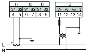
б) Однофазное подключение / Single-phase connection / Бір фазалық жалғау (1P2W, 1-TT, 1-TH)
