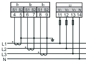
h) Трехфазное, четырехпроводное подключение / Three-phase, four-wire connection / Yш фазалык, төрт сымды жалғау (3P4W, 3-TT, 0-TN)
