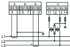
е) Трёхфазное, трёхпроводное подключение / Three-phase, three-wire connection / Үш фазалық, үш сымды жалғау (3P3W, 2-TT, 2-TH)
