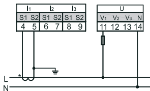
а) Однофазное подключение / Single-phase connection / Бір фазалық жалғау (1P2W, 1-TT, 0-TH)
