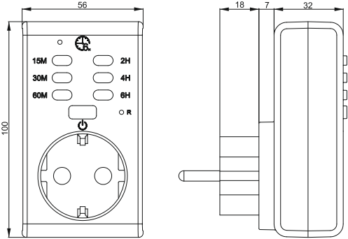
Габаритные размеры / Overall dimensions / Габариттік өлшемдері / Dimensiunile gabaritelor
