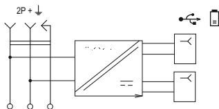
Рисунок 1 – Электрические схемы розеток / Figure 1 – Electrical diagrams of sockets / 1-сурет – Розеткалардың электр схемалары / Figura 1 – Schemele electrice ale prizelor
