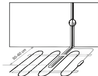
Рисунок 2 – Расположение датчика температуры / Figure 2 – Location of temperature sensor / 2-сურет – Температура бергішінің орналасуы / Figura 2 – Amplasarea senzorului de temperatură / ნახატი 2 – ტემპერატურის გადამწოდის განლაგება / 2-сურет – Температура сенсорунун жайгашкан жери / Расми 2 – Чойгиршавии сенсори ҳарорат / 2- rasm – Harorat datchigining joylashuvi
