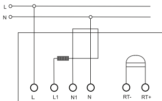
Рисунок 3 – Электрическая схема подключения / Figure 3 – Electrical connection diagram / 3-сურет – Электр қосылымының схемасы / Figura 3 – Schema electrică de conectare / ნახატი 3 – ჩართვის ელექტრული სქემა / 3-сურет – Электр туташуу диаграммасы / Расми 3 – Диаграммаи пайвасти барқ / 3 – rasm – Elektr ulanish sxemasi
