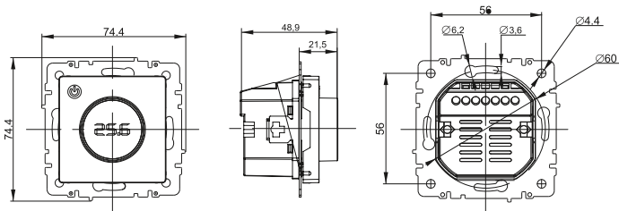
Рисунок 1 – Габаритные и установочные размеры / Figure 1 – Overall and installation dimensions / 1-сүрөт – Габариттік және орнату өлшемдері / Figura 1 – Dimensiunile generale și de instalare / ნახატი 1 – გაბარიტული და საყენებელი ზომები / 1-სურეტი – Көлем жана орнотмо өлшемдері / Расми 1 – Андозаи умумӣ ва насбӣ / 1-rasm – Umumiy va o'rnatish o'lchamlari
