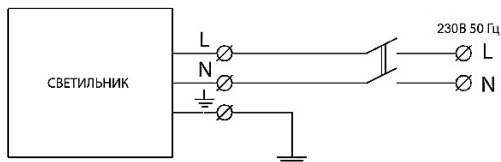
Рисунок 5 Схема подключения светильника
