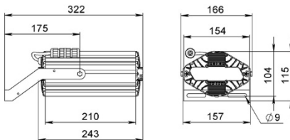
Рисунок 2 Общий вид светильника «L-lego II 55 banner» Поворотное крепление
