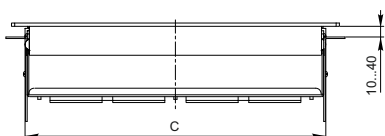
Рисунок 3 – Блок розеточный с односторонней крышкой / Figure 3 – Socket block with one-sided cover / 3 сурет – Бір жақты қақпақты розеткалы блок
