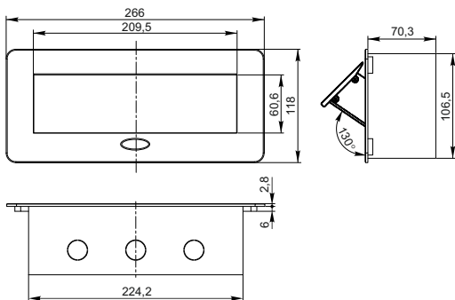
Рисунок 2 – Блок розеточный с выдвижной крышкой 6 модулей / Figure 2 – Socket block with retractable cover 6 modules / 2 сурет – 6 модульдің ысырмалы қақпақты розеткалы блогы (PM-BR51-06-O-KXX)
