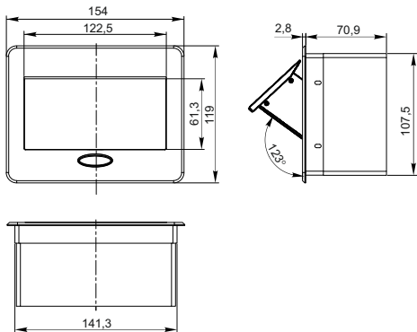
Рисунок 1 – Блок розеточный с выдвижной крышкой 4 модуля / Figure 1 – Socket block with retractable cover 4 modules / 1 сурет – 4 модульдің ысырмалы қақпақты розеткалы блогы (PM-BR51-04-O-KXX)
