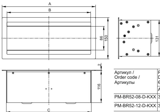
Рисунок 4 – Блок розеточный с двусторонней крышкой / Figure 4 – Socket block with double-sided cover / 4 сурет – Екі жақты қақпақты розеткалы блок
