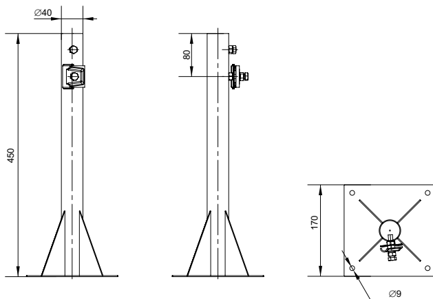
Рисунок / Figure 1 – Габаритные размеры / Overall dimensions
