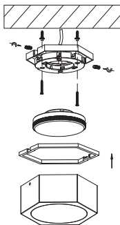
Рисунок 5 – Схема монтажа светильников типа 5204, 5304
